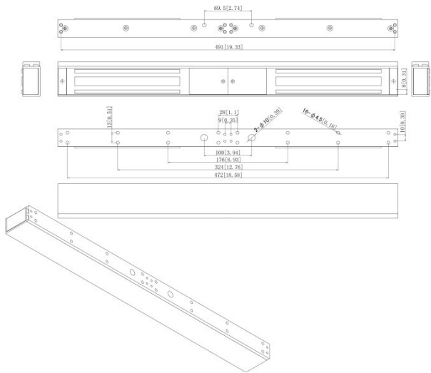
DHI-ASF280L-V1 Support de serrure magnétique
